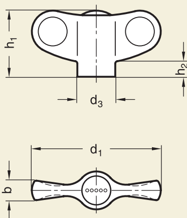
Form E mit Gewinde-Sackloch
