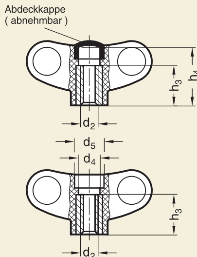
Form D mit Gewinde-Durchloch
